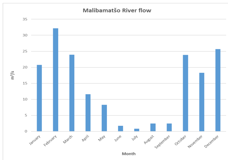
Fig 4.4 Malibamatšo river flow
