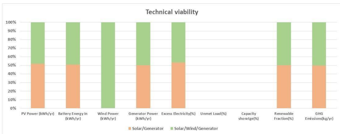
Fig 4.83 Technical values
